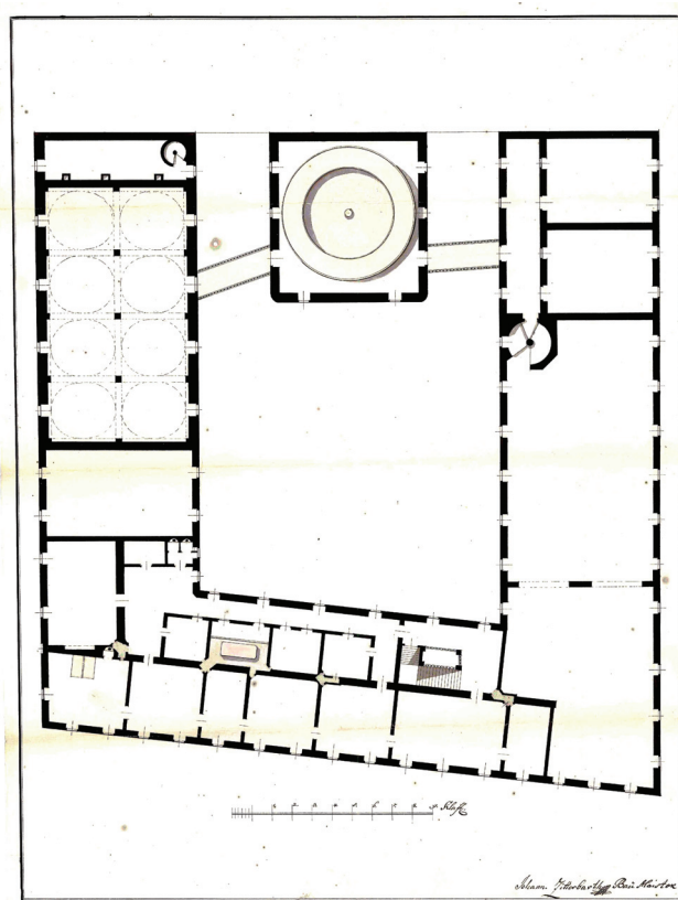
2. ábra. Mayerffy Serfözde, 1815, emeleti alaprajz (Forrás: [11] Budapest Főváros Levéltár 15.17.b.311 szb. 01393b)
