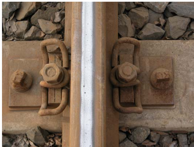
1. kép: Az Skl-12 típusú szorítórugóval szerelt, GEO alátételeztes, betonlajjas sínleerősítés felülnézetben
