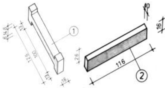
21. ábra A két típusú eloregyártott vasbeton elem (1-EA, 2-EL): alkotói a szilárd struktúrának és a rugalmas kivitelezett építményeknek
